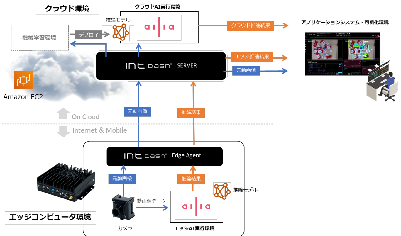
【ailiaSDK と intdash によるハイブリッドでリアルタイムな AI/IoT 環境構造図】
